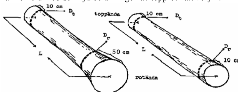
Figur 3. Måttställning.
